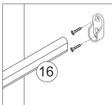
Установка штанги
