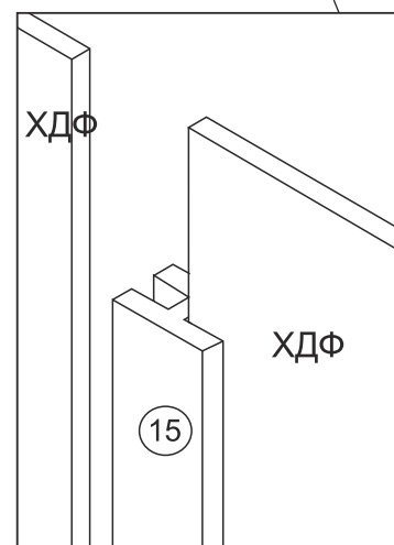
Монтаж ножки
